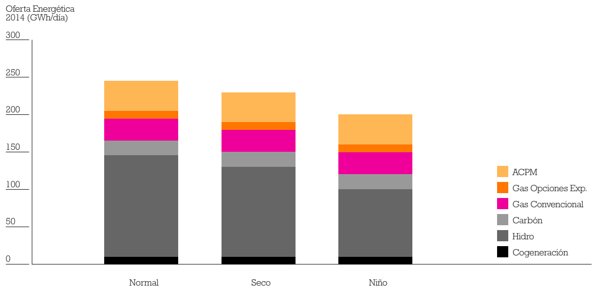
Gráfico 3.1. Oferta Energética del Sector Eléctrico en Colombia frente a la variación en la hidrología
